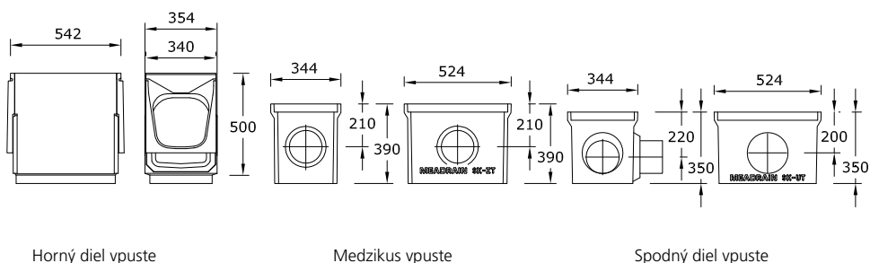
Horný diel vpuste
