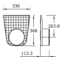
MEARIN Plus/Expert 300 čelná doska plná s odtokom DN200
