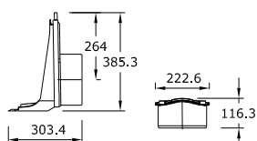
MEARIN Plus/Expert 300 čelná doska plná s odtokom DN200 pre bočné napojenie
